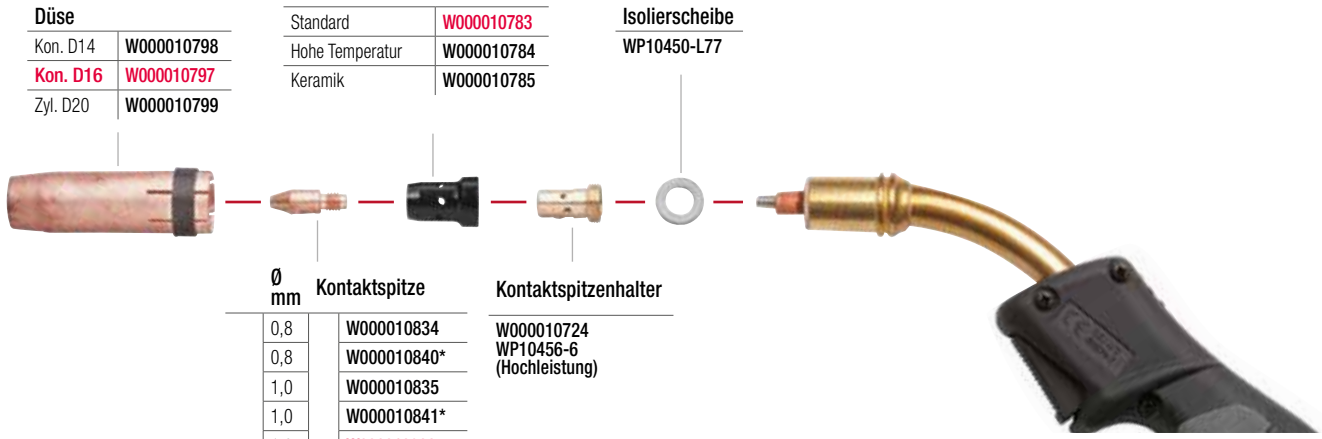
Isolierender Diffusor
